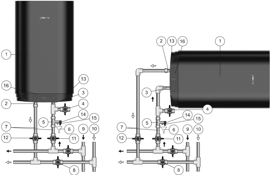
Abbildung 1. Anschlussdiagramm des Warmwasserspeichers an die Wasserversorgung
